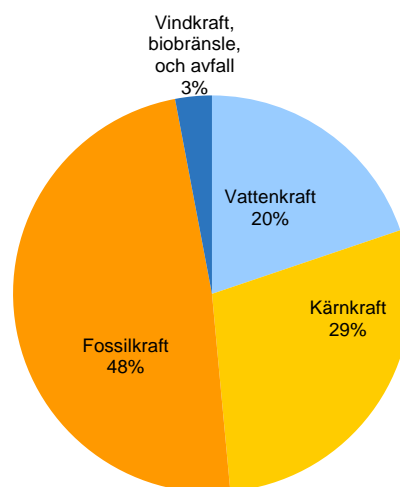
Elproduktion, Kv 2 2013 %
