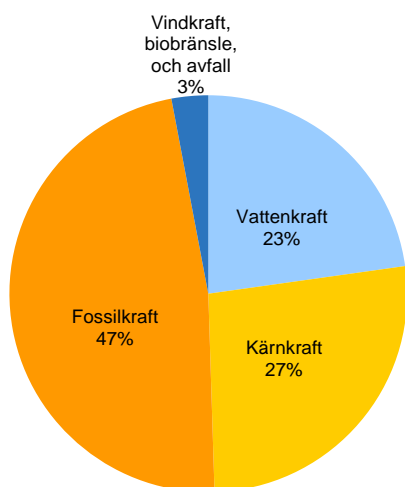
Elproduktion, Kv 2 2014 %
